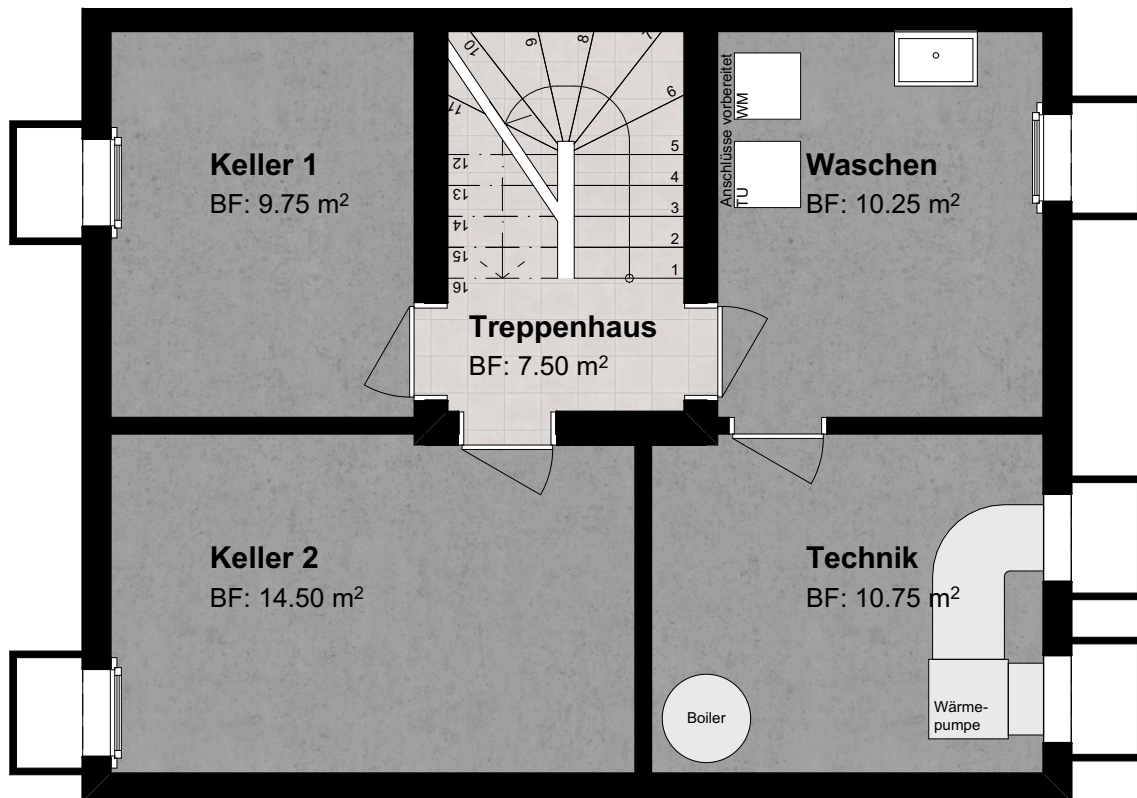
Haus B, Parzelle 1359
